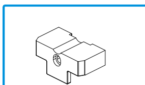
210307 TOPO LATERAL SUP. N°1 OS FLOW Utilizar com os aros laterais SO 08, 17 e 18 Parafuso M5x35 não incluído Material: ABS | Acabamento: Preto
