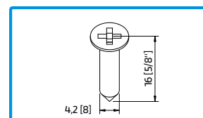
290077 PARAF. DIN7982 PH 4,2x16 INOX A2 Para fixar a peça magnética do Fecho suave magnético OS T Material: Inox | Acabamento: Inox
