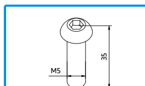
290118 PARAFUSO ISO7380 M5X35 INOX A2 Para fixar o Topo lateral sup. n°1 OS-Flow (Ref. 210307) Material: Inox | Acabamento: Inox
