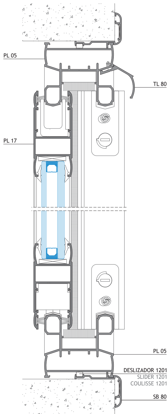
COM O PERFIL SB 80 WITH PROFILE SB 80 AVEC PROFIL SB 80
