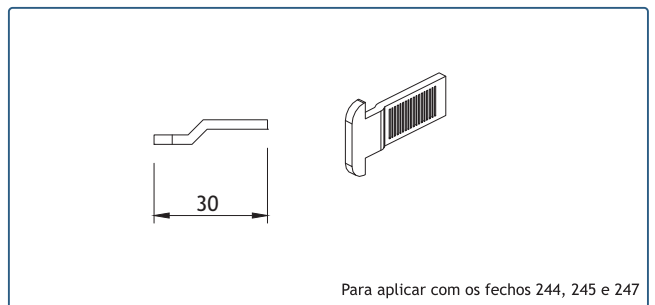
204723 GANCHO PL / TL
