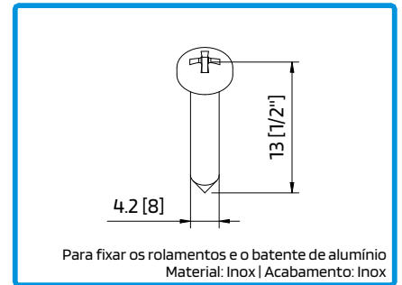
290111 PARAFUSO CQ 4,2x13 INOX A2
