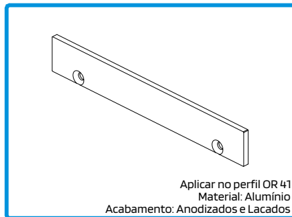
210106 TOPO OR 41 SILL END-CAP EMBOUT POUR SEUIL Aplicar no perfil OR 41 Material: Alumínio Acabamento: Anodizados e Lacados
