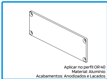
210105 TOPO OR 40 LINTEL END-CAP EMBOUT POUR LINTEAU Aplicar no perfil OR 40 Material: Alumínio Acabamentos: Anodizados e Lacados
