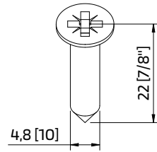
290170 PARAFUSO CX 7/8x10 INOX A2
