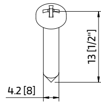
290111 PARAFUSO CQ 4,2x13 INOX A2
