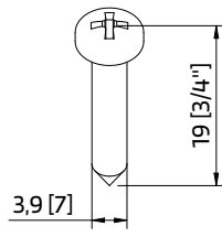
290063 PARAF. DIN 7981 3,9x19 A2
