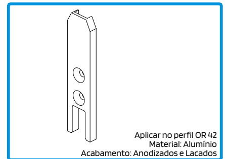
210229 TOPO FOLHA OR-PV Nº2 SASH END-CAP EMBOUT POUR VANTAIL Aplicar no perfil OR 42 Material: Alumínio Acabamento: Anodizados e Lacados
