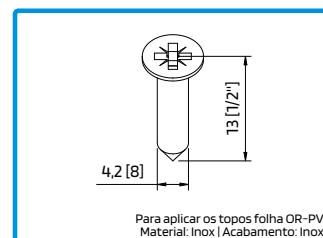
290061 PARAF. DIN7982 PH 4,2x13 INOX A2
