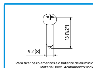
290111 PARAFUSO CQ 4,2x13 INOX A2
