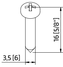
290729 PARAF PKI PH 5/8x6 CQ
