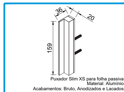
200057 PUXADOR FOLHA PASSIVA SLIM XS
