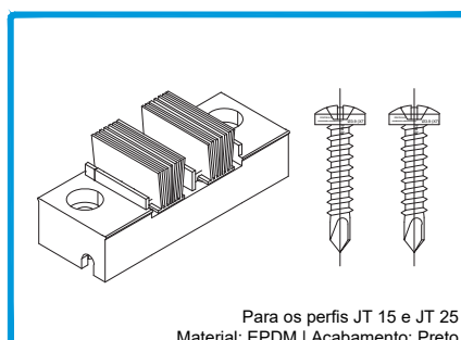
213303 CORTA VENTO JT FIXO
