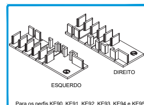
212223 CONJ. TOPOS INFERIORES RENOVATO
