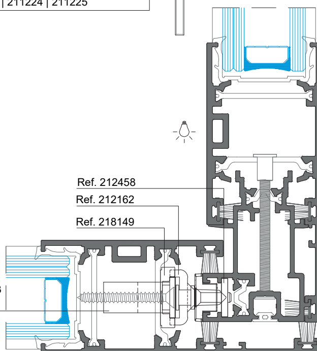
212455 CONJ. FIX. CONTRA-FECHO AL MULTIP. JT
