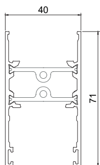
JT 63 Travessa inferior Lower transom | Traverse inférieur
