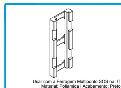
218149 CALÇO Nº2 P/ MULTIP. SOS JT
