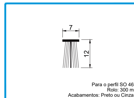
208593 PELÚCIA 7x12 STOP-FIN Cinza 208466 PELÚCIA 7x12 STOP-FIN Preto
