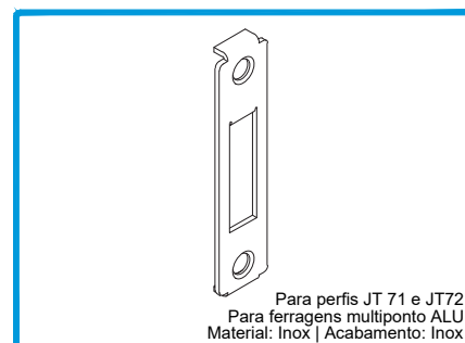
202331 CONTRA-FECHO Nº2 2F/90° ALU
