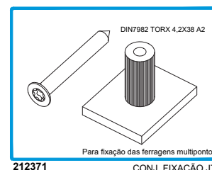
212371 CONJ. FIXAÇÃO JT
