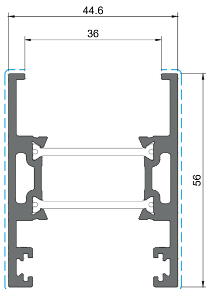
JT 60 Perfil lateral Lateral profile | Profilé latéral
