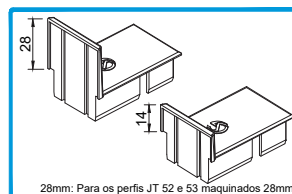
28mm: Para os perfis JT 52 e 53 maquinados 28mm 14mm: Para os perfis JT 52 e 53 maquinados 14mm Material: Poliamida | Acabamento: Preto
