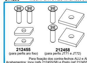
212455 CONJ. FIX. C.-FECHO AL MULTIP. JT 212458 CONJ. FIX. C.-FECHO 2F/90º JT
