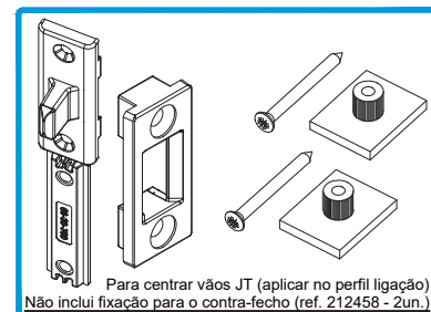
212162 CONJ. CENTRADOR P/ FERRAGEM JT PERFIL LIG.
