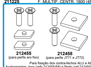
212455 CONJ. FIX. C.-FECHO AL MULTIP. JT 212458 CONJ. FIX. C.-FECHO 2F/90° JT
