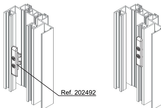
FERRAGEM MULTIPONTO SOT MULTIPOINT HARDWARE | SERRURE MULTIPONT
