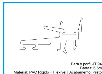
208349 JUNTA CENTRAL 2195 JT FIXO
