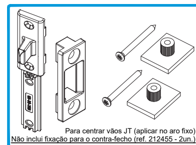
212161 CONJ. CENTRADOR P/ FERRAGEM JT
