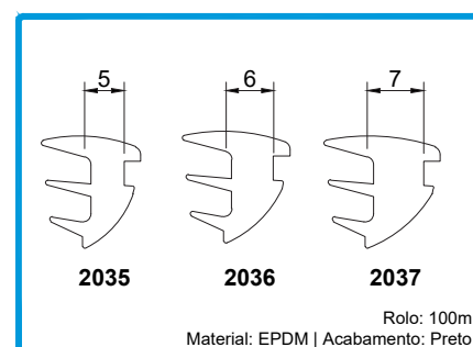
208196 JUNTA DE CUNHA 2035 208215 JUNTA DE CUNHA 2036 208904 JUNTA DE CUNHA 2037
