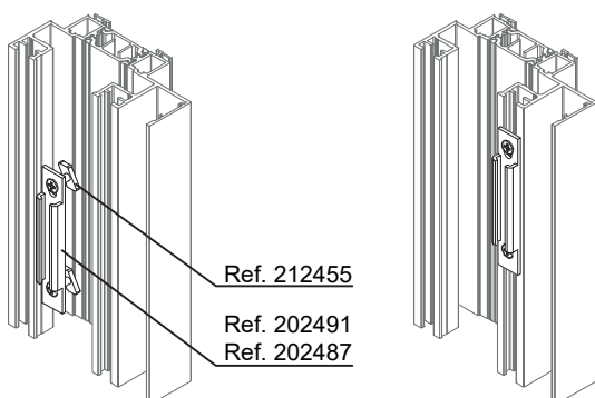
FERRAGEM MULTIPONTO SOS MULTIPOINT HARDWARE | SERRURE MULTIPONT
