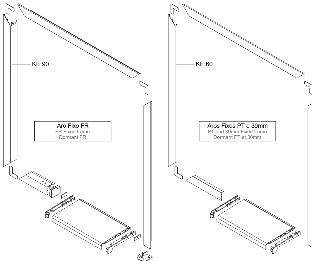
212223 CONJ. TOPOS INFERIORES RENOVATO
