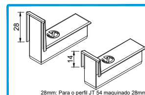
28mm: Para o perfil JT 54 maquinado 28mm 14mm: Para o perfil JT 54 maquinado 14mm Material: Poliamida | Acabamento: Preto
