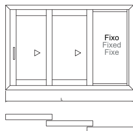
Corte | Cut | Coupe D-D
