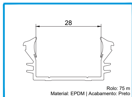
208477 JUNTA VIDRO U 1028 CX 28MM JT
