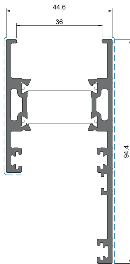
JT 70 Perfil lateral canto 90° 90° Corner lateral profile | Profilé latéral d'angle à 90°
