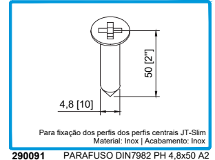
290091 PARAFUSO DIN7982 PH 4,8x50 A2
