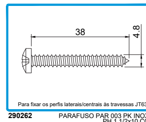
290262 PARAFUSO PAR 003 PK INOX PH 1 1/2x10 CQ
