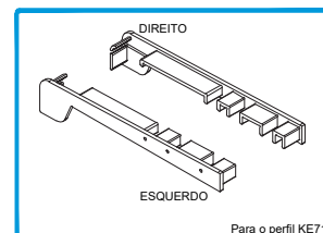
212221 CONJUNTO TAPA TOPOS KE 71
