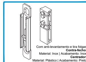
202491 CONTRA-FECHO ANTI-LEV. MULT. 202487 CENTRADOR JT P/G-FECHO AL M.
