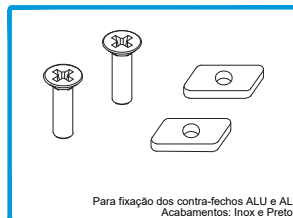
212455 Para fixação dos contra-fechos ALU e AL Acabamentos: Inox e Preto CONJ. FIX. CONTRA-FECHO AL MULTIP. JT
