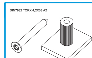
212371 CONJ. FIXAÇÃO JT Para fixação das ferragens multiponto
