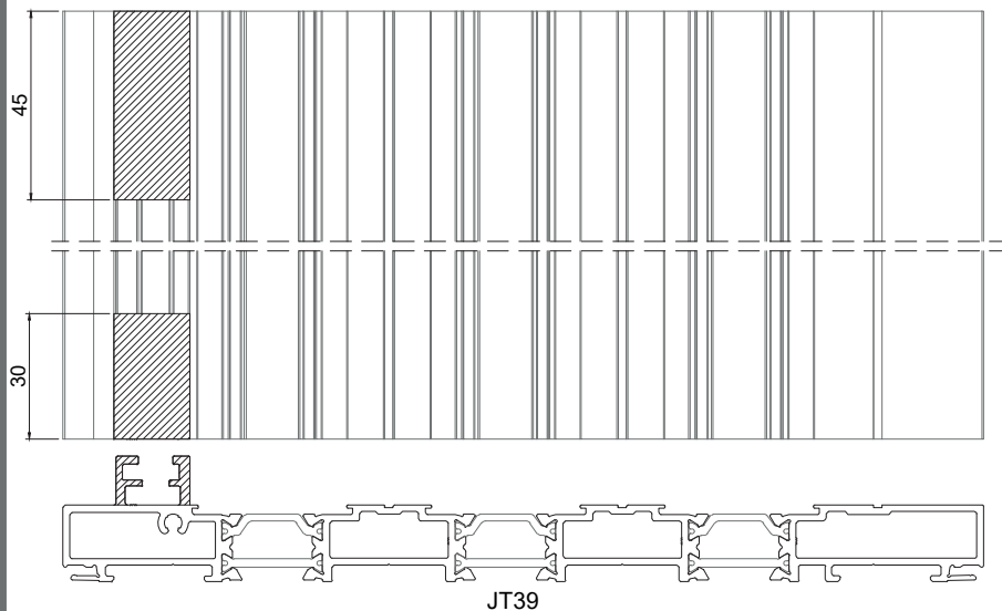
JT39
