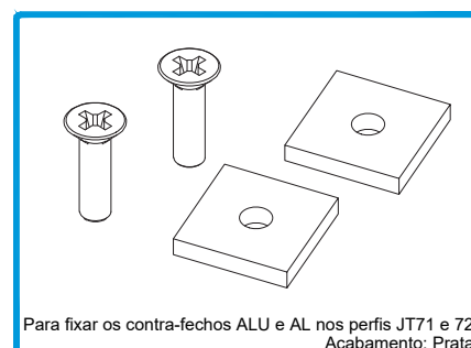
212458 CONJ. FIX. CONTRA-FECHO 2F/90° JT
