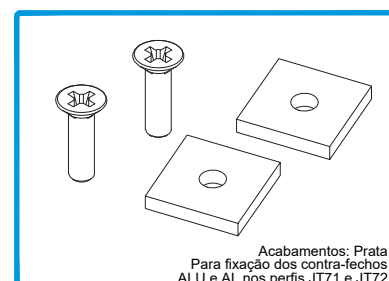
212458 CONJ. FIX. CONTRA-FECHO 2F/90° JT
