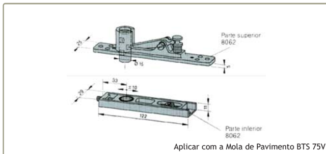
227111 PIVOT SUPERIOR VAI-VEM 8062
