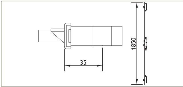
201010 FECHADURA DE 3 PONTOS EM U 7799x35
