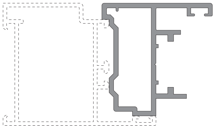
MONTAGEM ASSEMBLY MONTAGE
