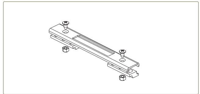
280005 TESTA PARA FECHADURA PS Nº2
