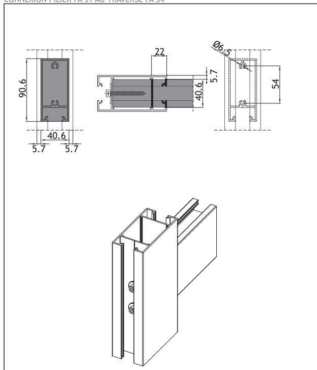
LIGAÇÃO MONTANTE PA 31 À TRAVESSA PA 34 CONNECTION COLUMN PA 31 TO TRANSOM PA 34 CONNEXION PILIER PA 31 AU TRAVERSE PA 34
