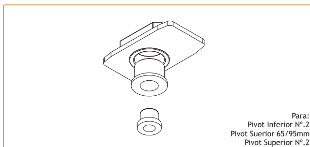
TOPO PIVOT Nº.6 PARA PA 41
