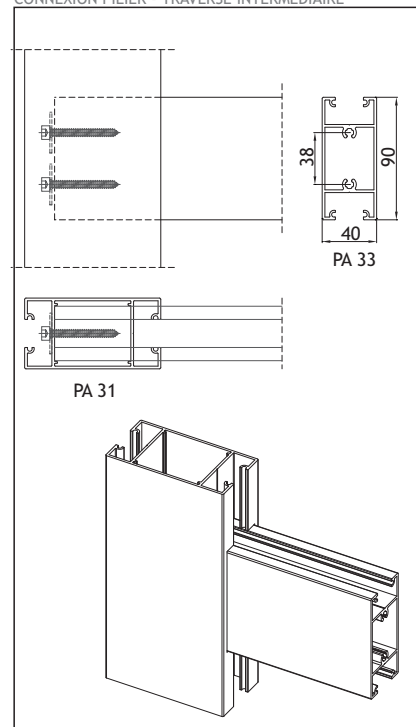
LIGAÇÃO MONTANTE - TRAVESSA INTERMÉDIA CONNECTION COLUMN-INTERMEDIATE TRANSOM CONNEXION PILIER - TRAVERSE INTERMÉDIAIRE
