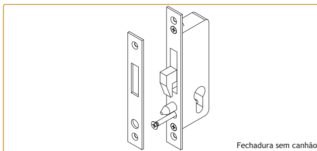
FECHADURA DE GANCHO SEM CILINDRO 9796
