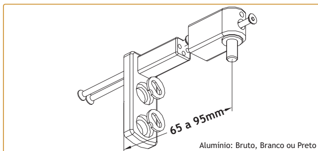
227123 PIVOT SUPERIOR Nº.3 65/95mm ALUMÍNIO Alumínio: Bruto, Branco ou Preto
