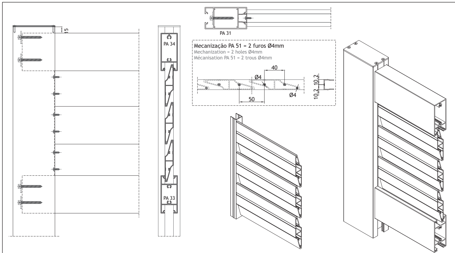
APLICAÇÃO DAS LÂMINAS PA 50 PA 50 BLADES APPLICATION APPLICATION DES LAMES PA 50
