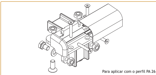
Para aplicar com o perfil PA 26
