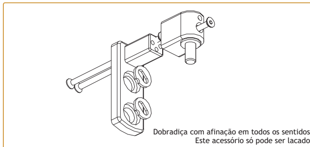
202164 DOBRADIÇA C/REGULAÇÃO PA 24000
