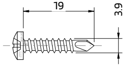
290472 PARAF. AT/PF CQ 3.9x19 A2
