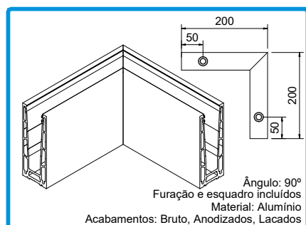
213032 CANTO 90° EXTERIOR AV 24
