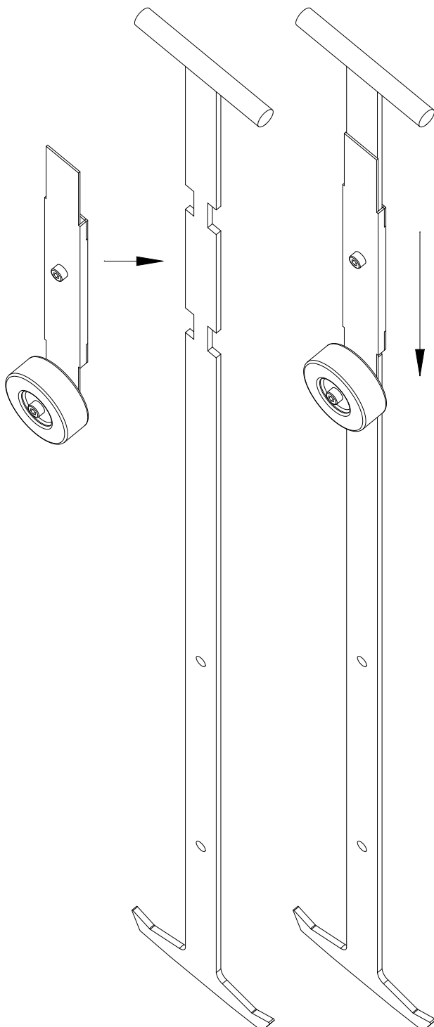
228222 FERRAMENTA P/ APLICAÇÃO DE JUNTAS AV
