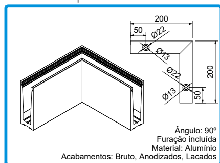
213020 CANTO 90° INTERIOR AV13
