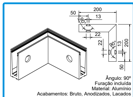
213023 CANTO 90° EXTERIOR AV14
