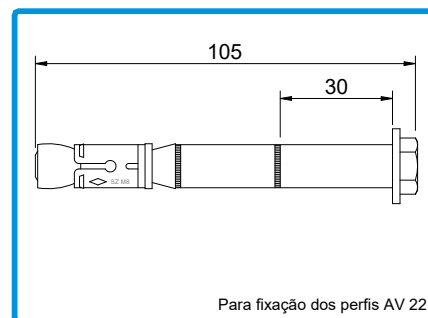
218098 BUCHA AÇO ZINC. AV SZ-S 12-30
