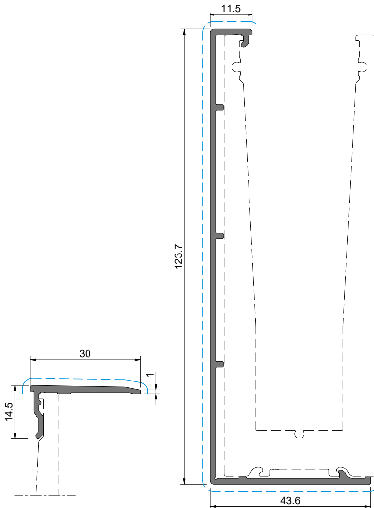
AV 05 Capa Cover | Capot
