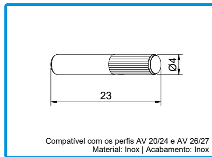
299157 VEIO 4MM P/ ALINHAMENTO AV
