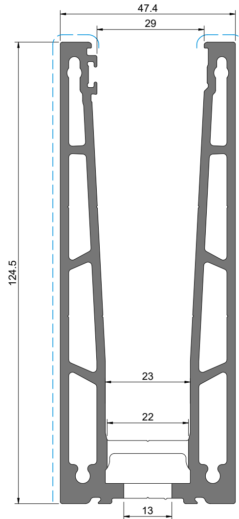
AV 24 Com furações inferiores With inferior milling Avec fraisage inférieur
